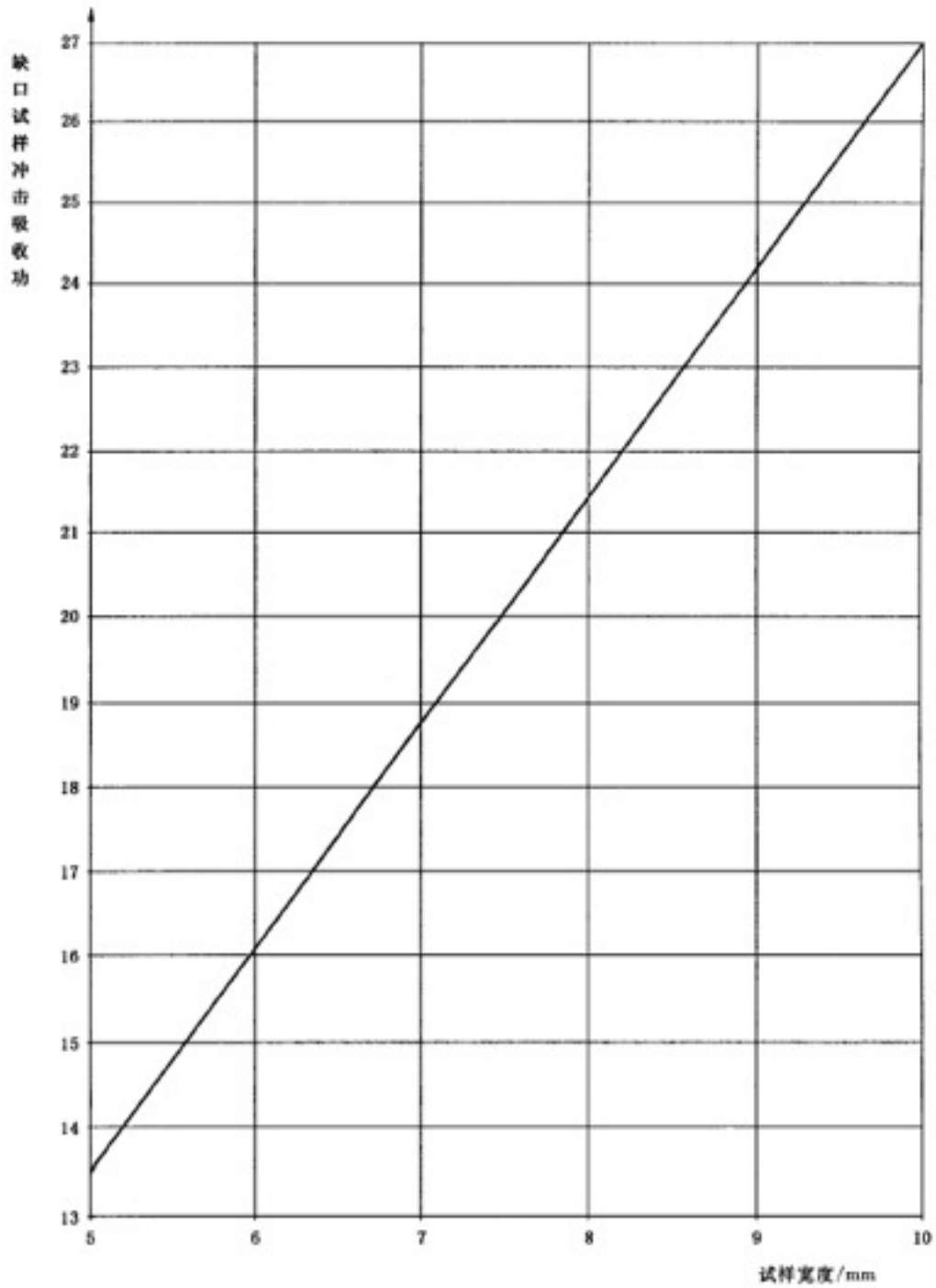
图中文字翻译：缺口试样冲击吸收功—поглощенная работа на удар пробы выреза 试样宽度/проба—ширина пробы/проба
